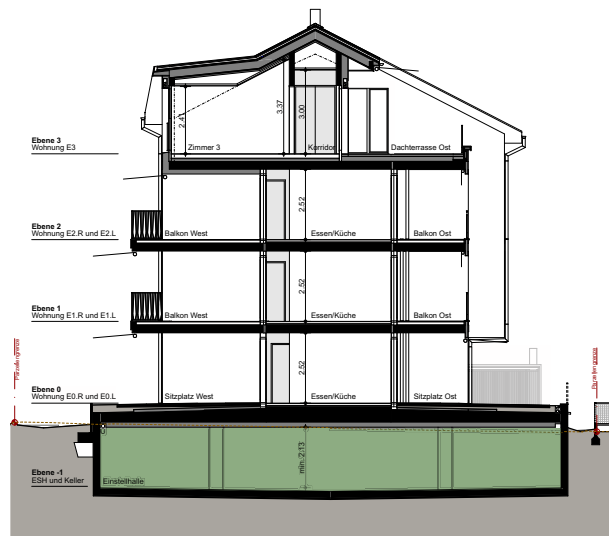
Schnitt «A»
